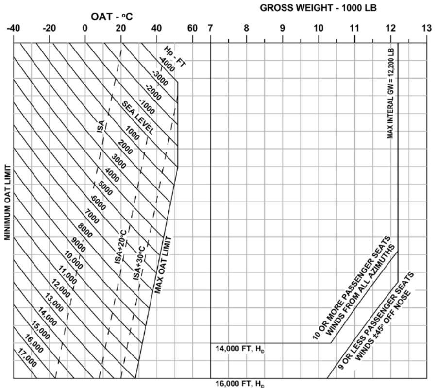
IGE Hover WAT Limitation
